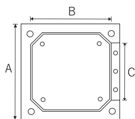
Terminal 終尾式
