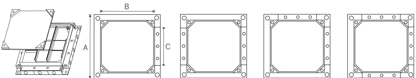
4 way 四通式
