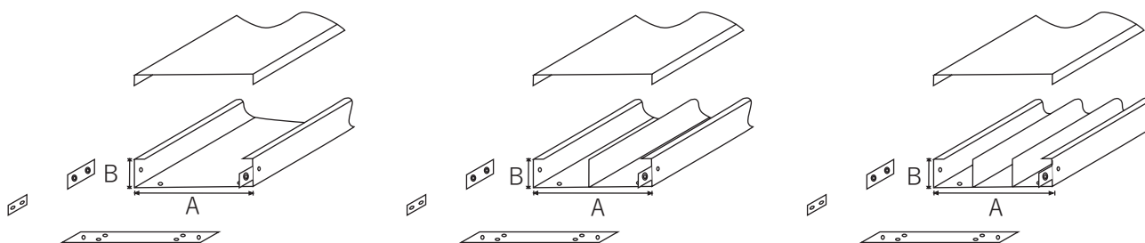
Standard type 標準型
