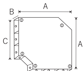
Flat elbow 平面曲
