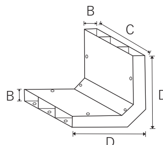
Vertical elbow 垂直曲
