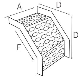
External Bend 外曲型
