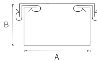
Clip Fix 彈夾蓋型
